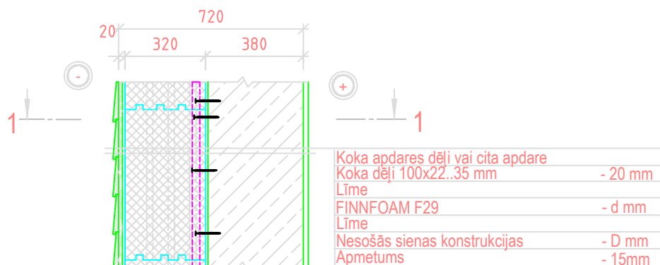
legriezums 1-1
