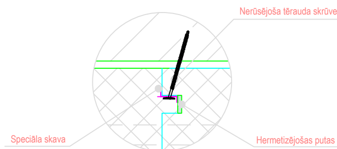
Detaļa A Mērogs 1:5
